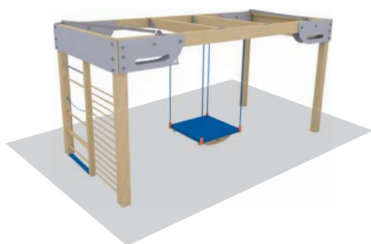
Variante 22 Sistema completamente indipendente Dimensioni: 500 x 228 x 273h
