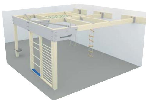
Variante 23 Sistema montato su un lato della parete, con pilastri indipendenti su un lato; Dimensioni: 500 x 442 x 273h
